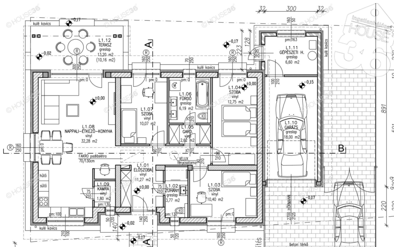
Alaprajz
