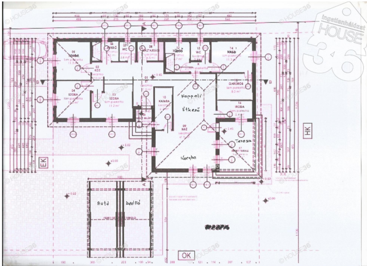
Alaprajz
