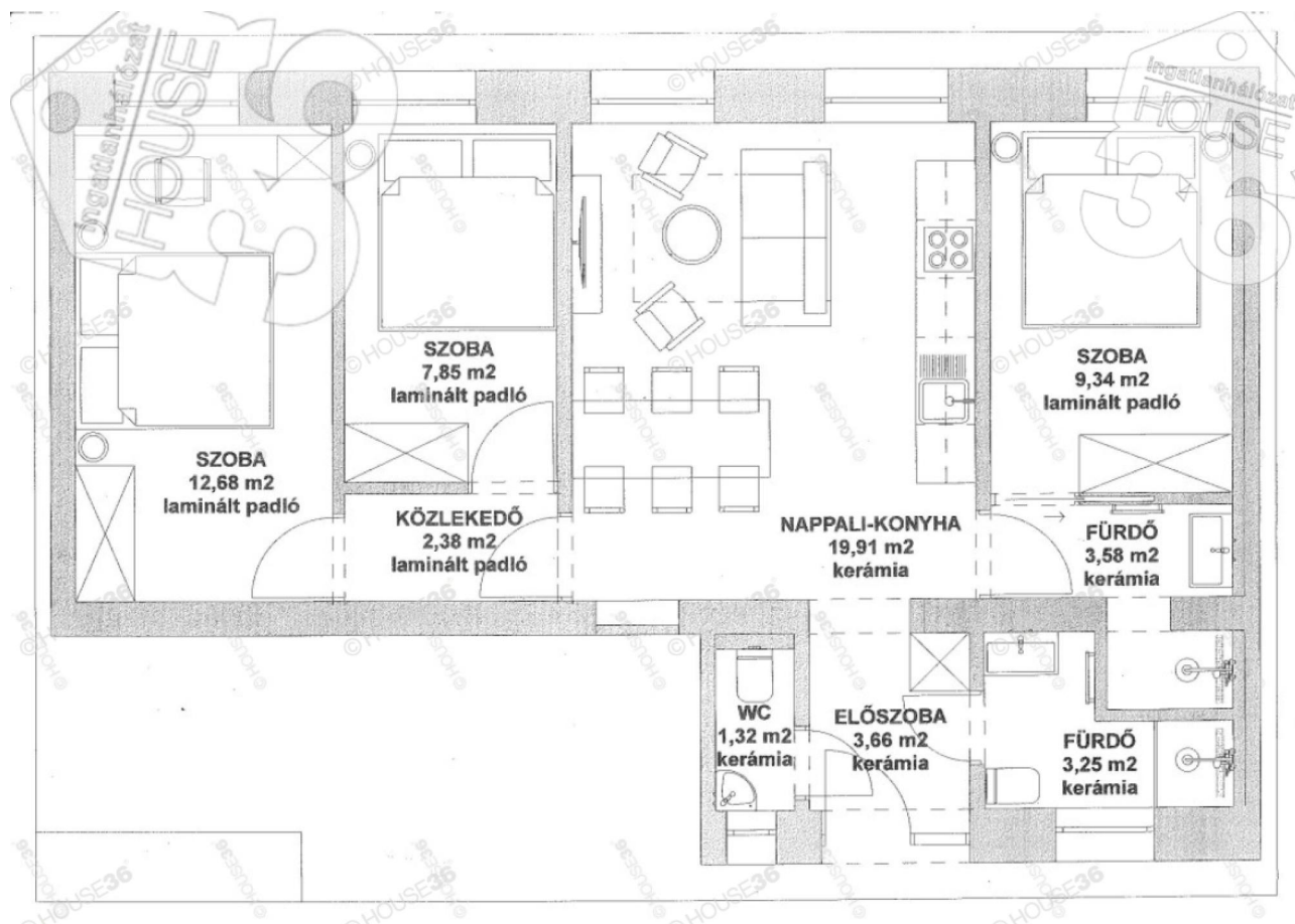
Alaprajz
