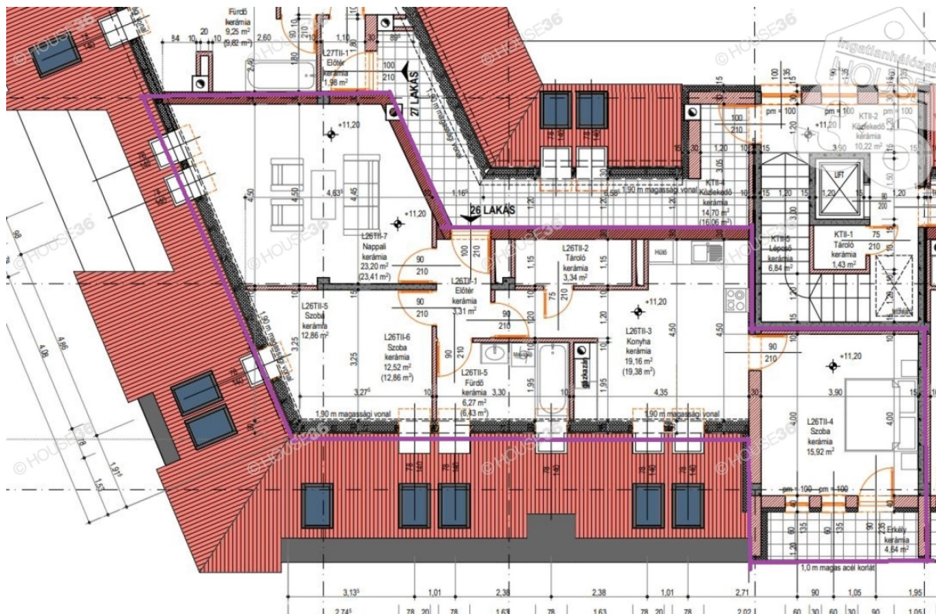
Alaprajz
