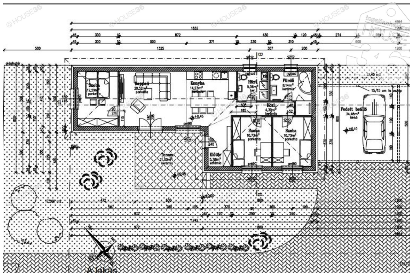
Alaprajz
