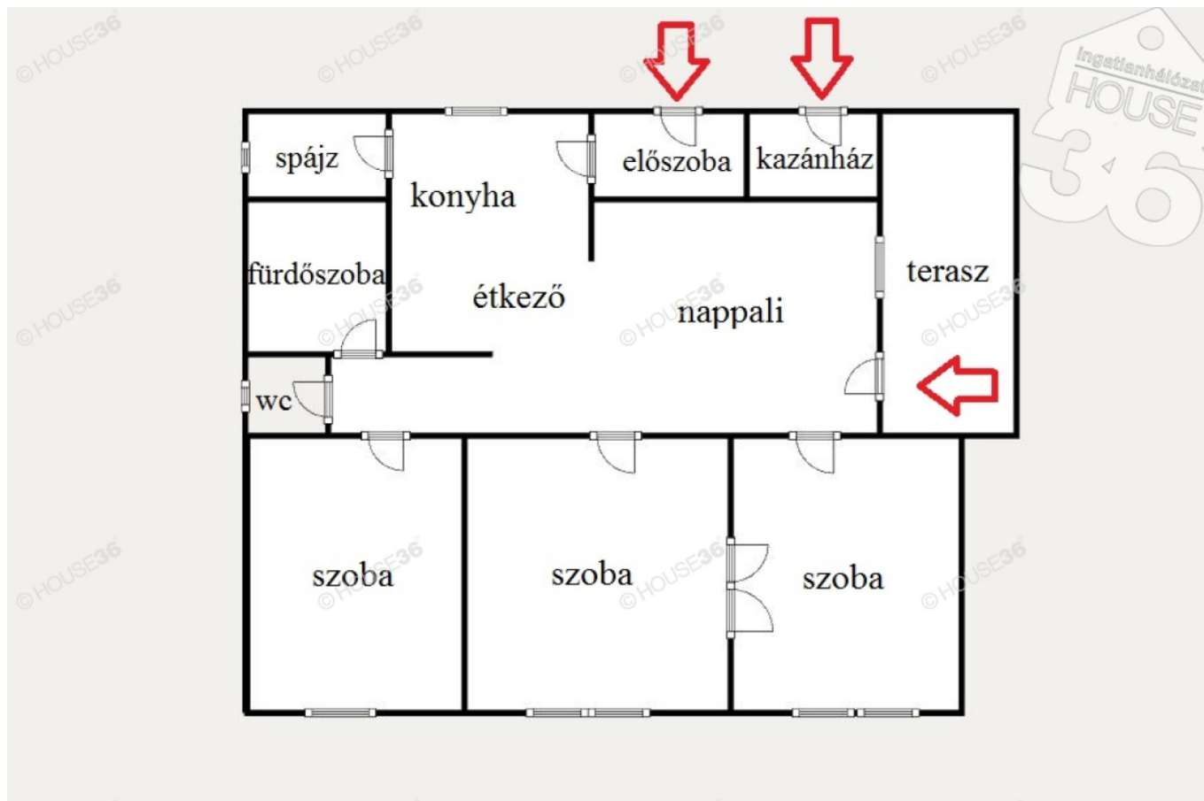
Alaprajz
