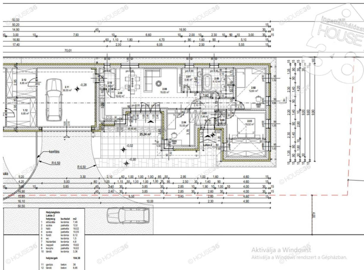
Alaprajz
