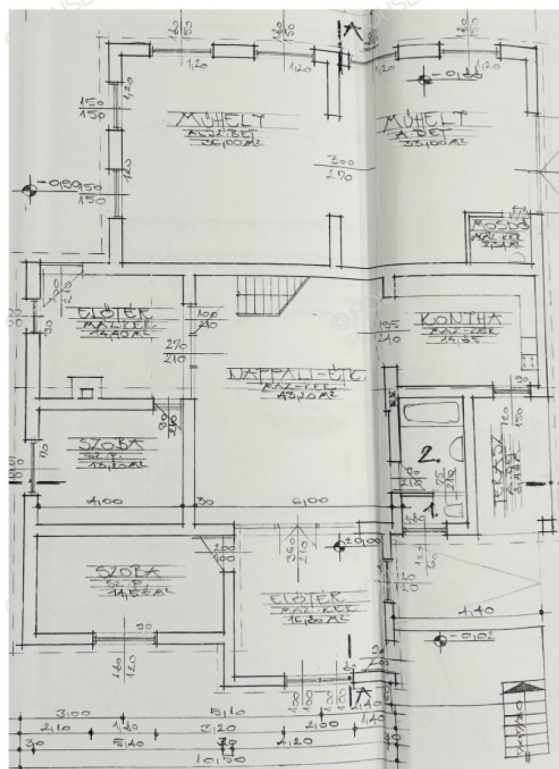
FÖLDSZINT ALAPRAJZ
