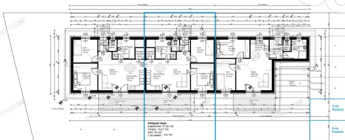
FÖLDSZINTI ALAPRAJZ M= 1: 100
