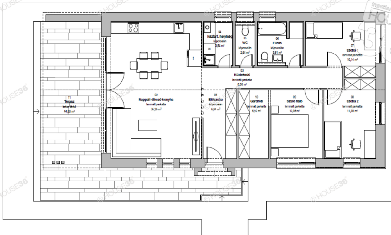
Alaprajz
