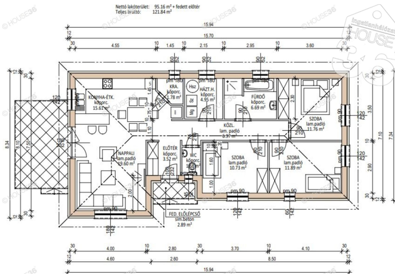
Alaprajz
