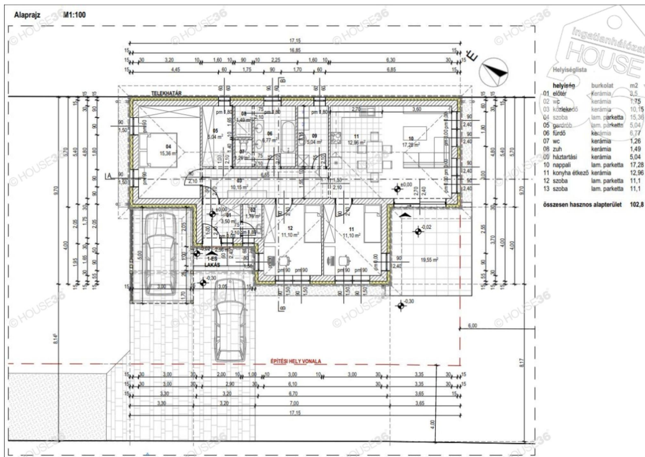
Alaprajz
