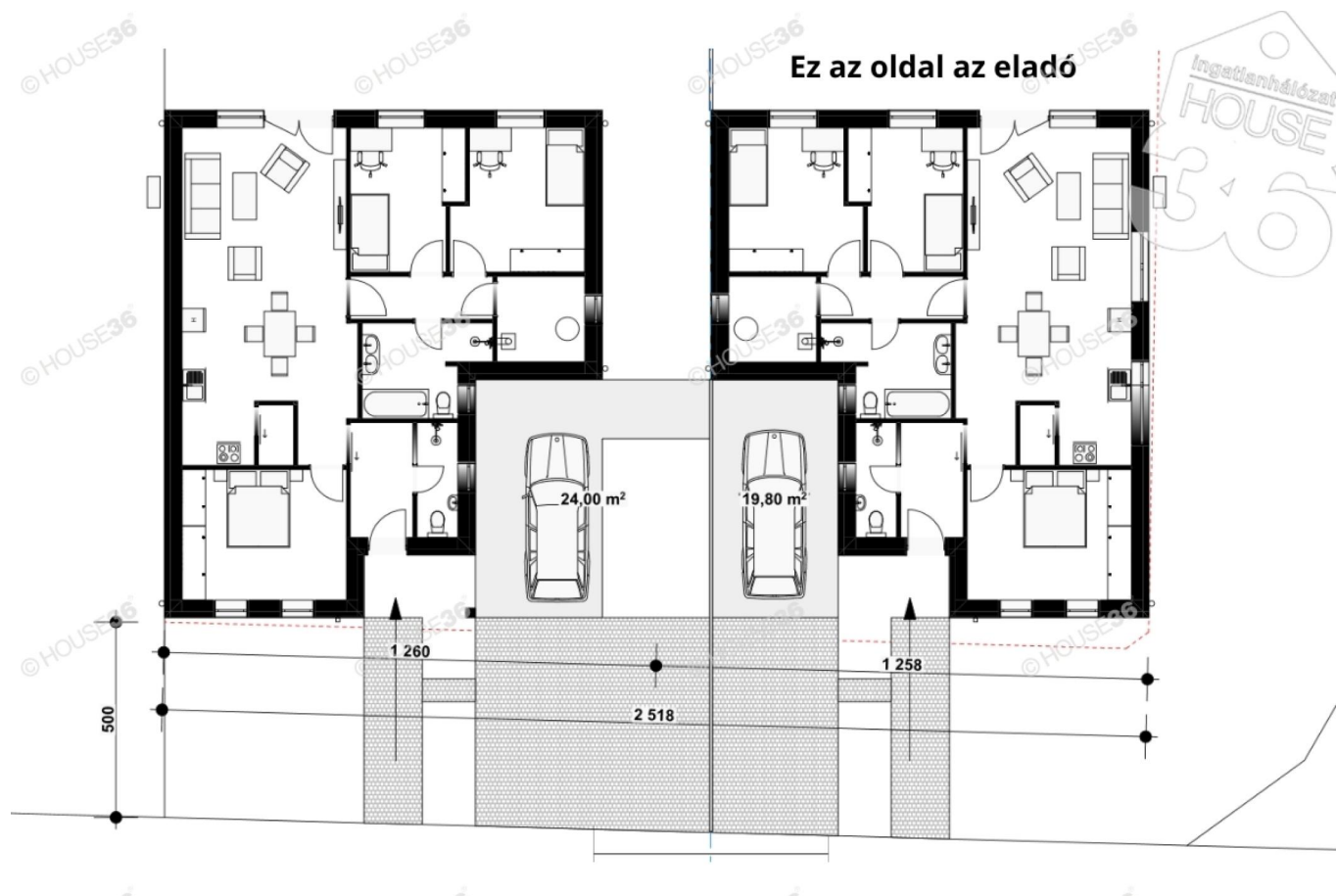
Alaprajz
